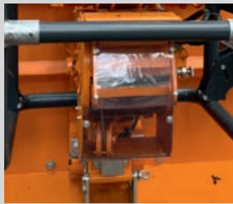
Seilspulung Rückholwinde
